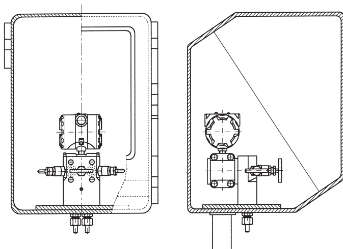
Beispiel für die Montage eines 3-fach Ventilblockes im Schutzkasten direkt auf der Bodenplatte
