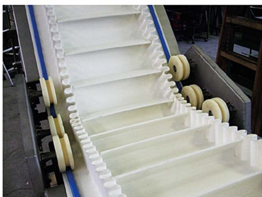
Bande de transport: bord ondulé avec des crampons
